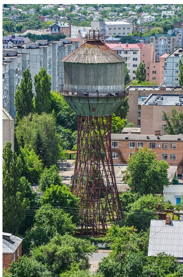
Шуховская водонапорная башня, начала XX века
